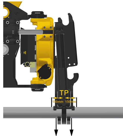
Afbeelding45. Maximale zwaartepuntverschuiving 150mm
