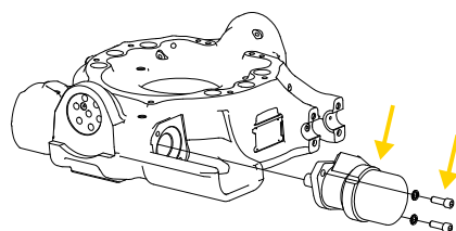
Afbeelding36. Verwijder de motor.
